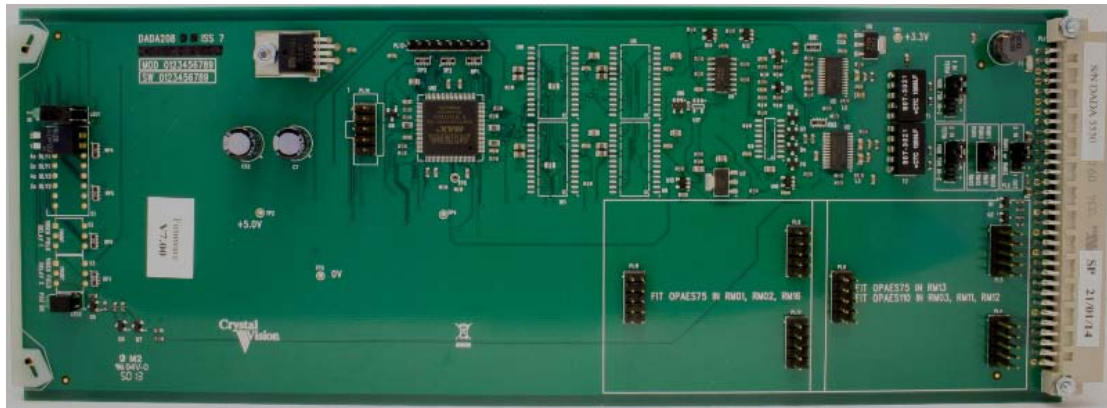
DADA208 dual digital audio DA
