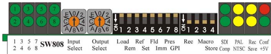
SW808 card edge
