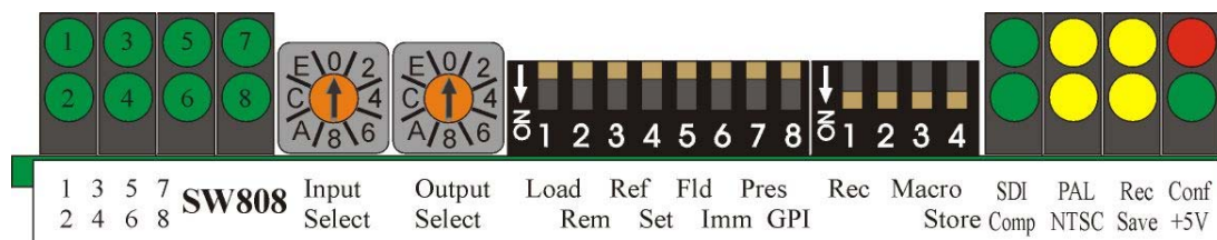
SW808 status LEDs
