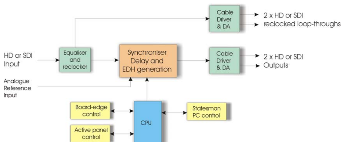
SYN HD block diagram
